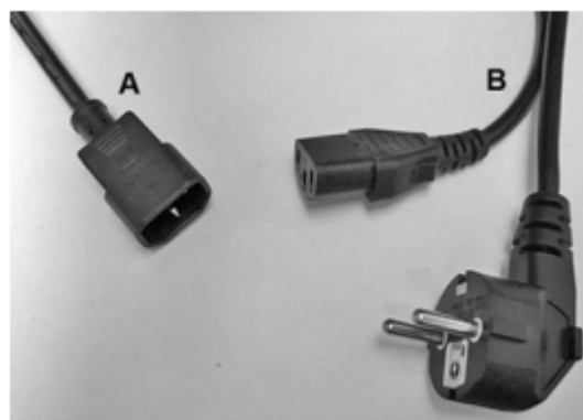
Bild 10 A = festangeschlossenes Kaltgerätekabel B = 5 m Kaltgeräte-Anschlusskabel
