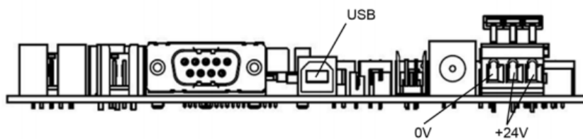
Bild 98 Seitenansicht CCTalk-Interface
