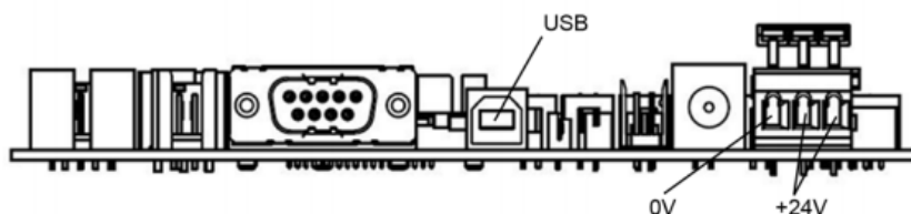
Bild 98 Seitenansicht CCTalk-Interface
