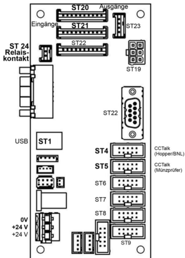
Bild 97 CCTalk-Interface CCT910
