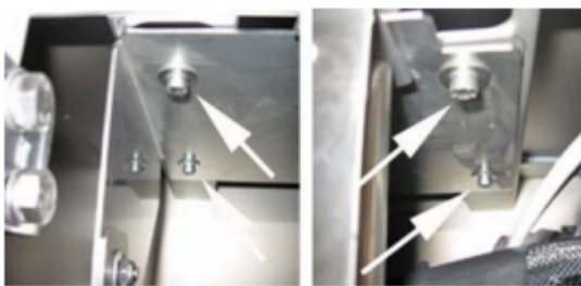
Bild 58 Schrauben links und rechts lösen.
