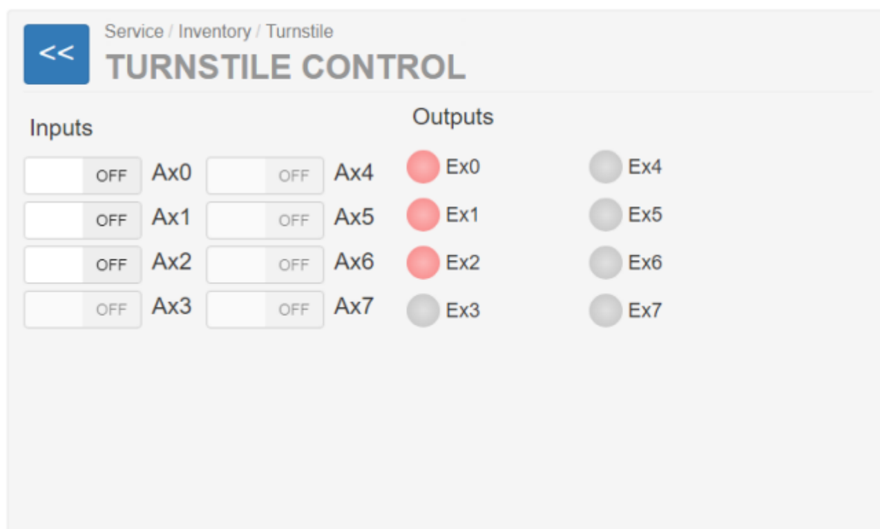
Bild 53 Steuer-Bildschirm Drehkreuz
